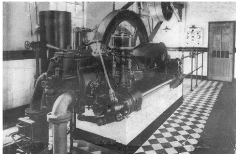
Een Deutz Zuiggas-Motor, die tot 1965 in gebruik was bij C&S.
