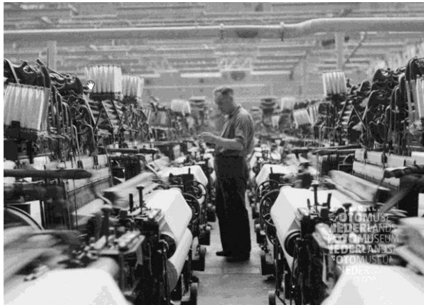
Interieur van textiel fabriek in Twente. (foto Ned. Textielmuseum)
